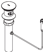
Assemblage du Drain
