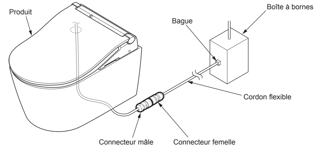
Exemple de connexion d'alimentation électrique
