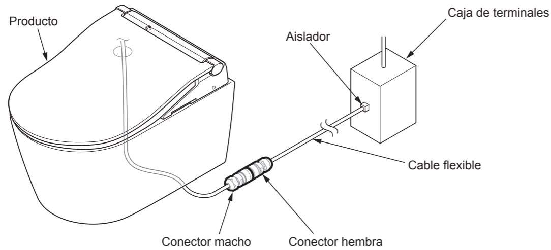
Ejemplo de conexión de la alimentación
