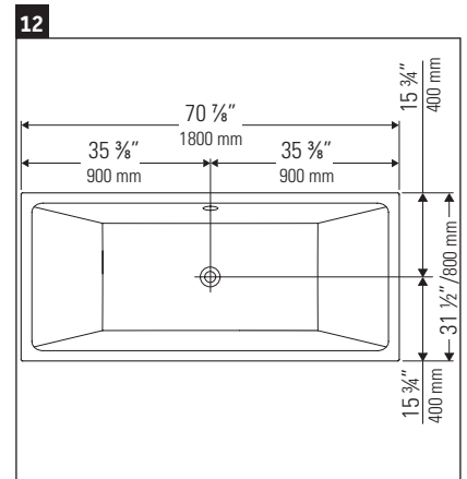
Medidas para Vero Air.
