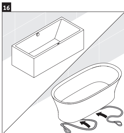
> Deslizar las correas por debajo de la bañera.
