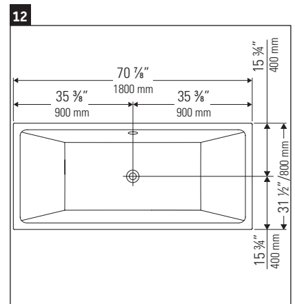
Dimensions pour Vero Air.
