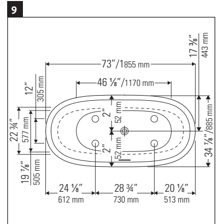
Dimensions pour Cape Cod.
