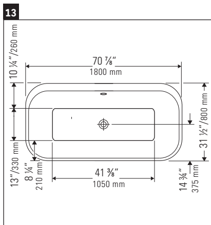
Medidas para Happy D.2 Plus.
