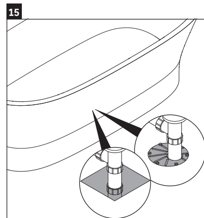
> Retirar las ayudas de instalación. > Conectar la bañera al sistema de desagüe.
